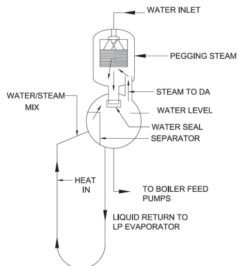
DEAERATOR IN HRSG SERVICE
