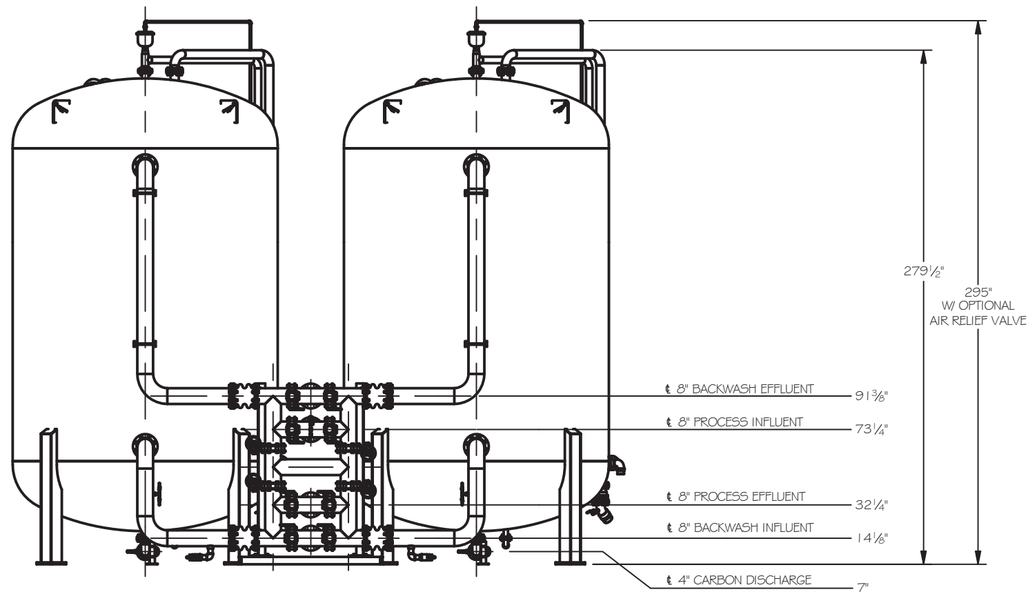
ELEVATION
