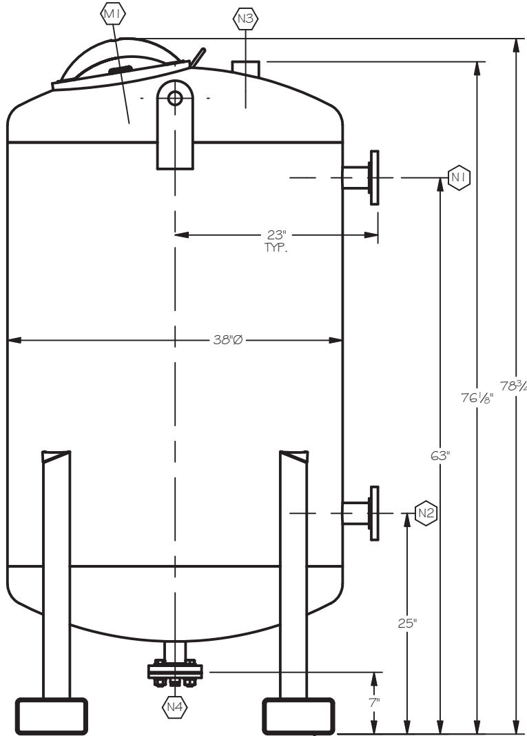
ELEVATION
